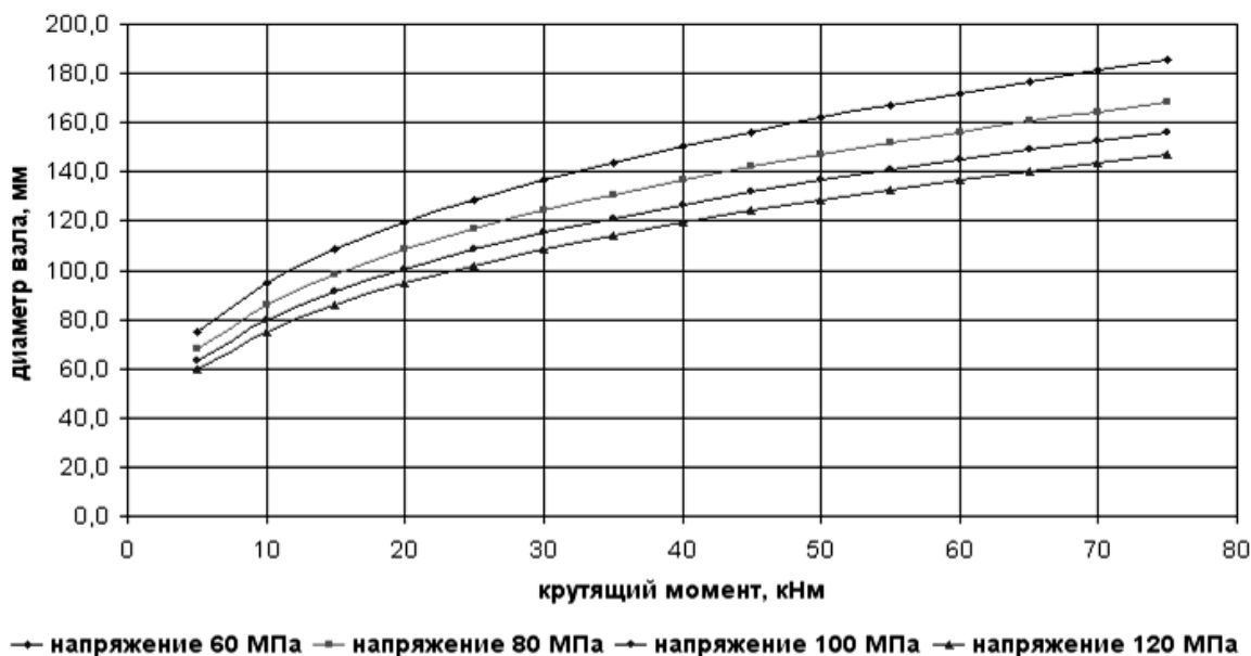
Рисунок 41 – Графики семейства кривых расчетного диаметра вала от величин крутящего момента и допускаемых напряжений
