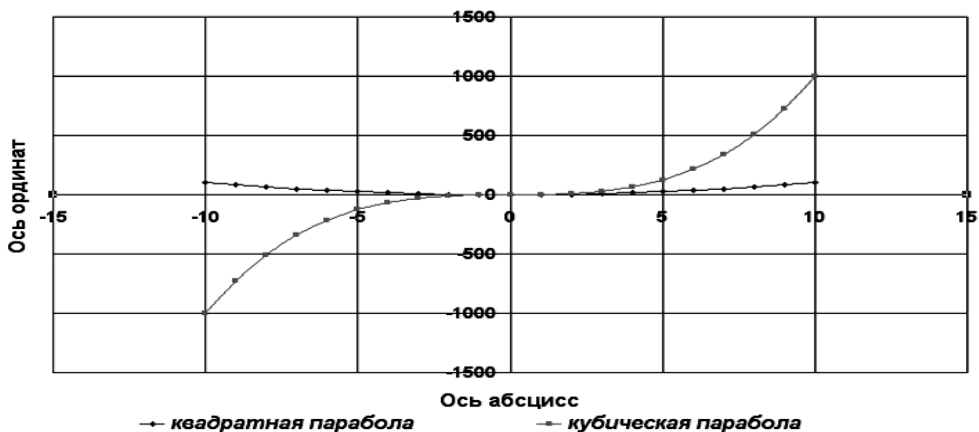
Рисунок 39 – Квадратная и кубическая параболы
